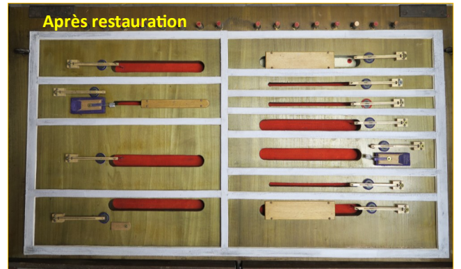
Joints d'étanchéité entre le sommier et la table
